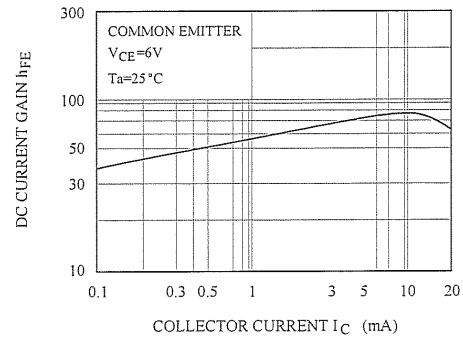
h_{FE} - I_C
